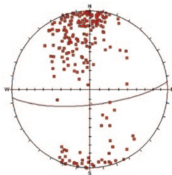
Abb. 6: Schieferungsflächen aus dem Tauernfenster mit einem Durchschnittswert von 174/74 (Schmidt'sches Netz, untere Halbkugel, 218 Daten).
