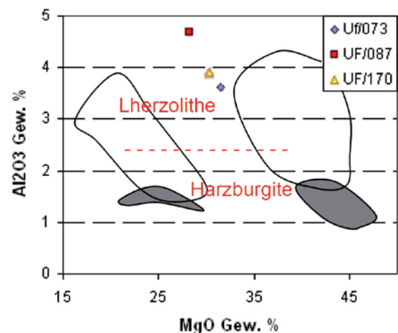
Abb. 18: \text{MgO} - \text{Al}_2\text{O}_3 Diagramm für ultramafische Gesteine der Penninischen Einheiten (ungefüllte Flächen: Ochsner, graue Felder: Stubachtal – Melcher et al., 2002) und den drei Proben (UF/073, UF/087, UF/170) aus dem Serpentinittkomplex (Schönberg-Spitz).
