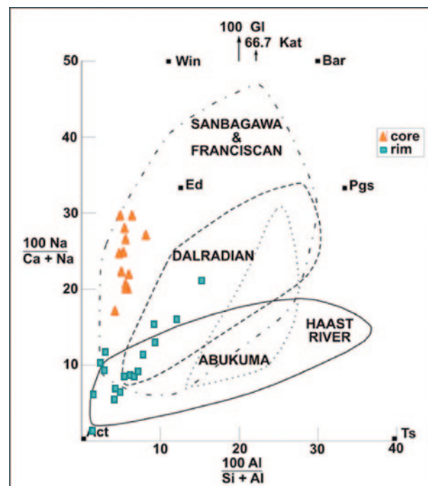
Abb. 17: Amphibole aus dem Grünschiefer: 100\text{Na}/(\text{Ca} + \text{Na}) – 100\text{Al}/(\text{Si} + \text{Al}) Diagramm von Laird and Albee (1981). Kern, Rand. Nach der Klassifikation von Leake et al. (2004) handelt es sich im Kern um Aktinolith und randlich um Magnesiohornblende.
