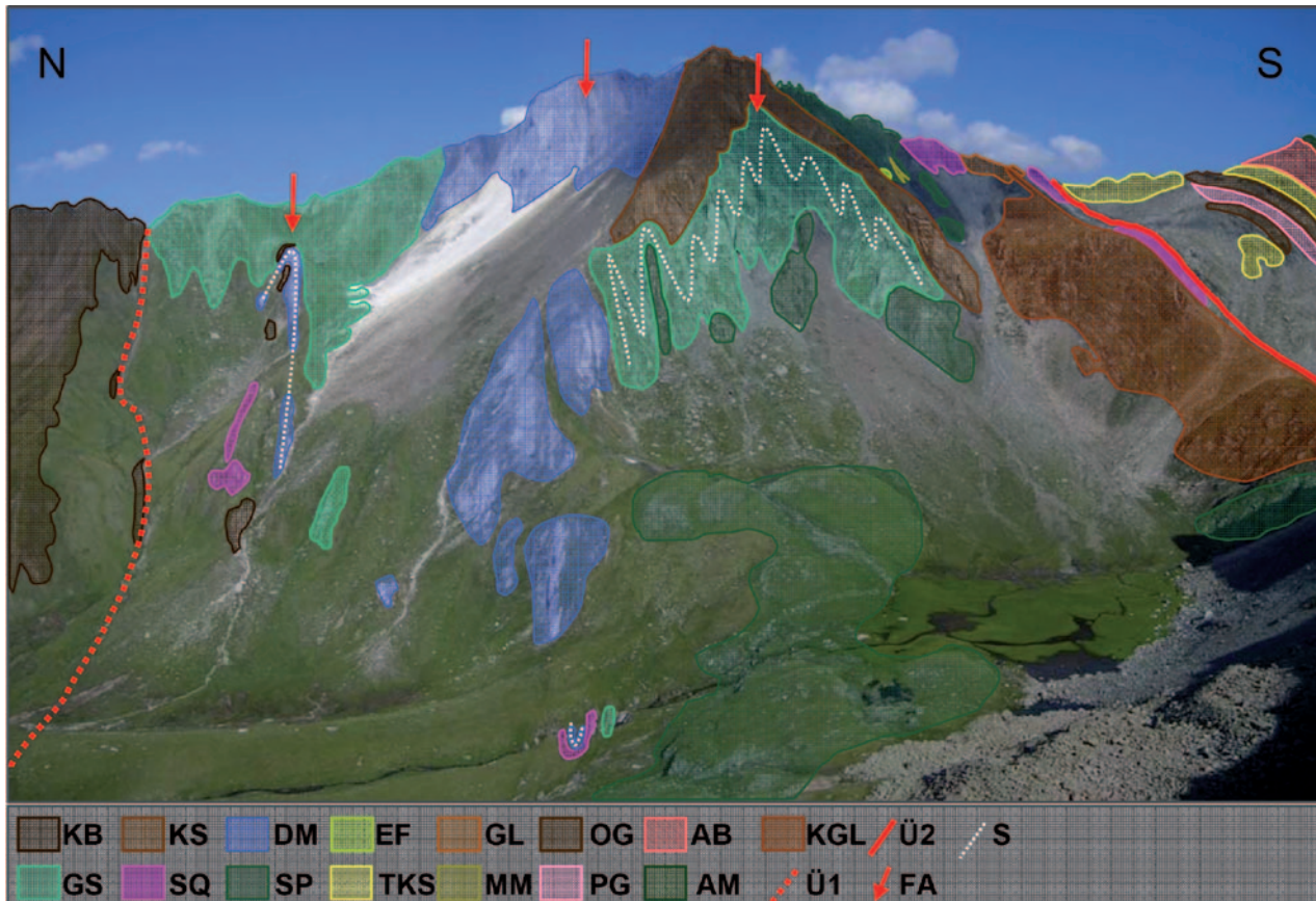
Abb. 2: Übersicht der Lithologien im Gelände am Schwarzspitz (Poinland) mit dem Übergang Bündnerschiefer – Serpentinithkomplex (Ü1) und Serpentinithkomplex – Ostalpin (Ü2). Die Falten streichen E-W, wobei die Faltenachsen (FA) steil nach Osten abtauchen; im Bild sind die verfalteten Schieferungsflächen (S) der Grünschiefer und Dolomitmarmore angedeutet. Links: die Bündnerschiefer mit Kalkglimmerschiefer und Schwarzphyllit (KB); Bildmitte: Serpentinithkörper mit Grünschiefern (GS), Dolomitmarmor (DM), Kalkglimmerschiefer (KS), Epidotfels (EF), Talk-Karbonat – Schiefer (TKS), Serpentinith (SP), Serizit-Quarzit (SQ), Glimmerschiefer (GL), kalkreicher Glimmerschiefer (KGL); Rechts: Metamergel (MM), Orthogneis (OG), Paragneis (PG), Albitblasten-Schiefer (AB), Amphibolit (AM)
