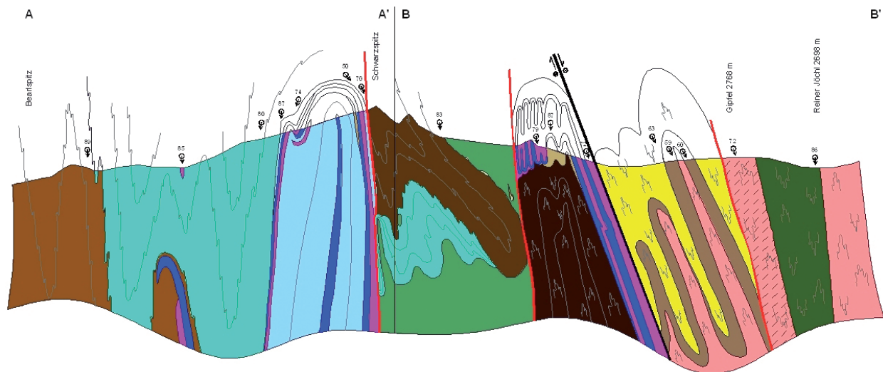
Abb. 4: Das geologische Profil (Spur A – A' und B – B' in Abbildung 3) verläuft in etwa Nord-Süd über den Bearispitz, den Schwarzsipz, den Gipfel 2768 m bis zum Reiner Jochl und ist in dieser Abbildung nicht maßstabsgetreu dargestellt (Legende für die Lithologien siehe Abbildung 3).
